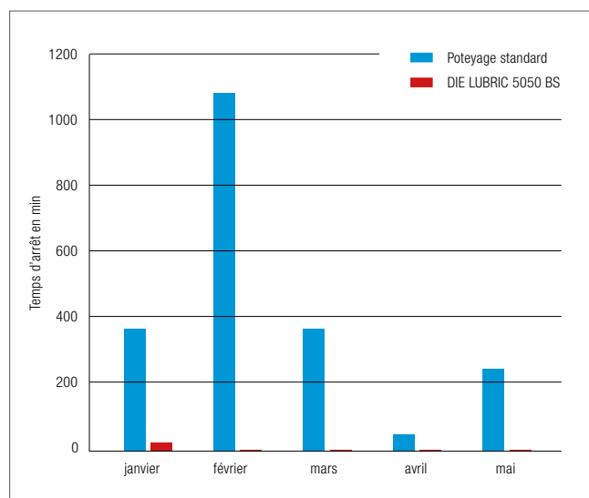
Temps d'arrêt de la machine lié au colmatage des buses
